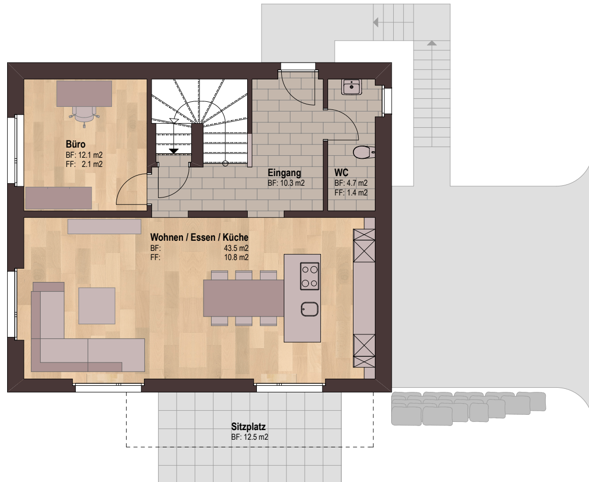
Erdgeschoss
