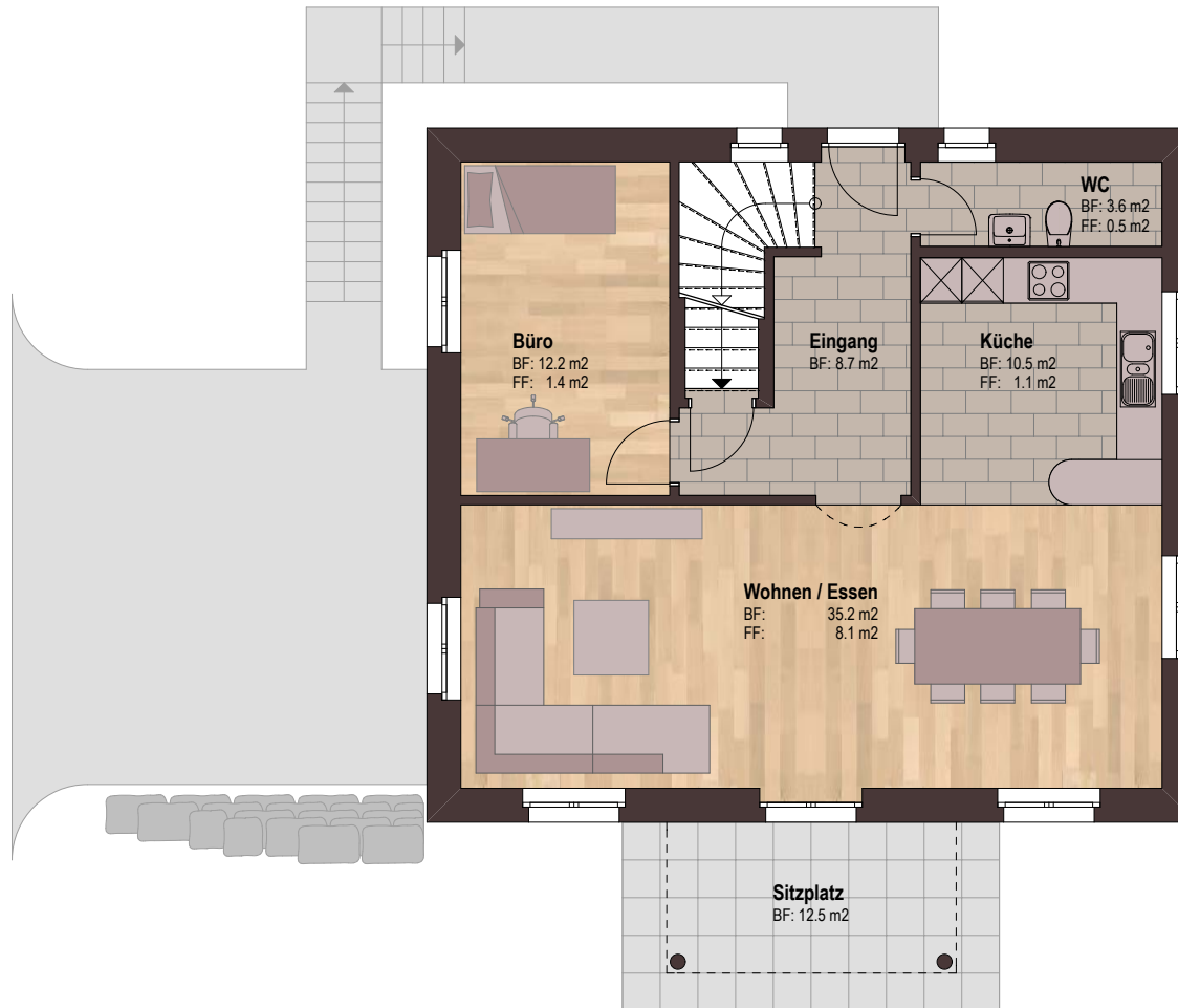
Erdgeschoss
