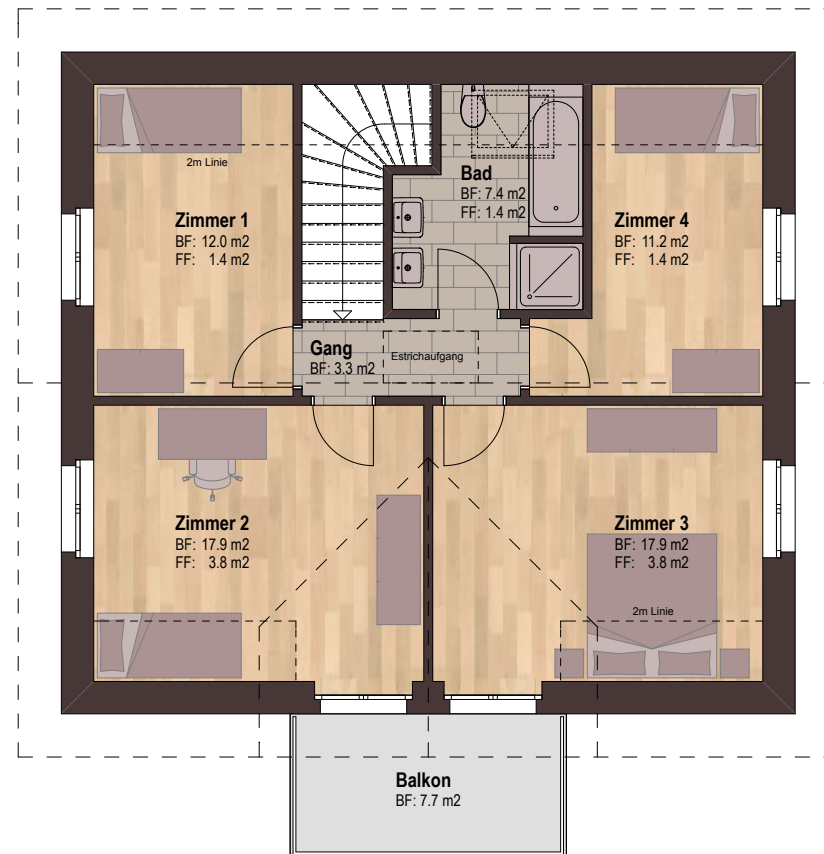
Obergeschoss 4 Zimmer
